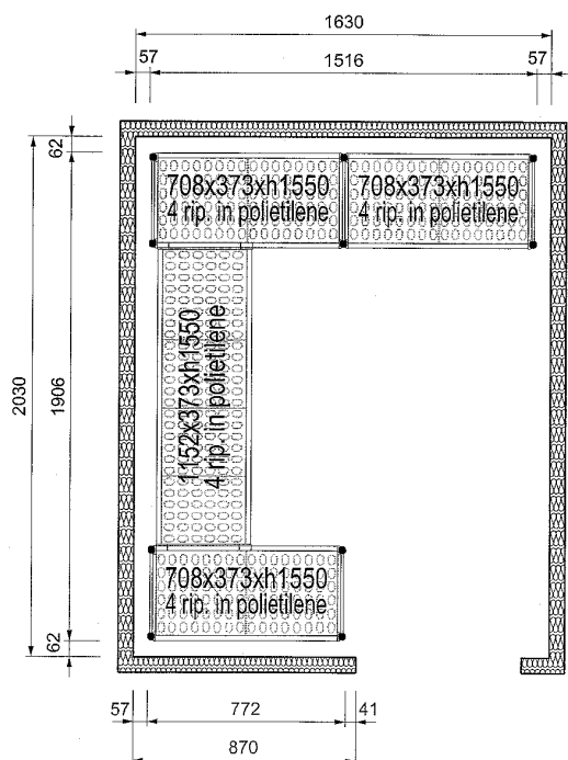
Boven aanzicht
